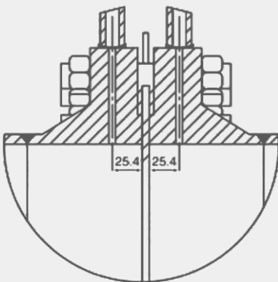
法兰取压
