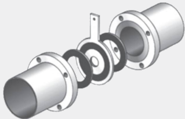
典型孔板装配
